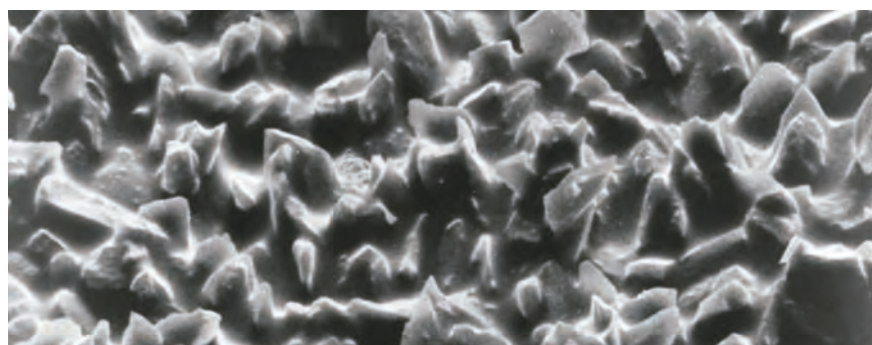
Imagen microscópica de grano abrasivo ST 5000, ampliación de aprox. 1000 aumentos
