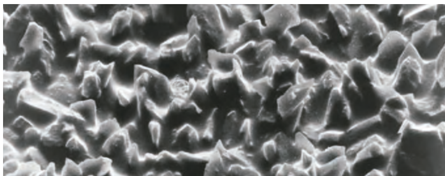
Imagen microscópica de grano abrasivo ST 5000, ampliación de aprox. 1000 aumentos
